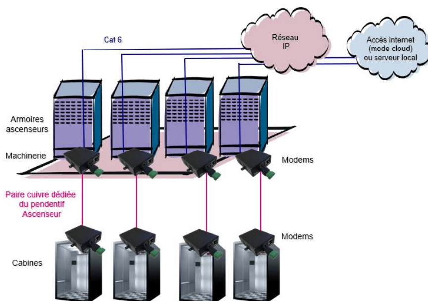
Exemple d'architecture pour 4 cabines
