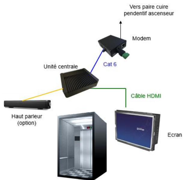
Schéma d'architecture ascenseur
