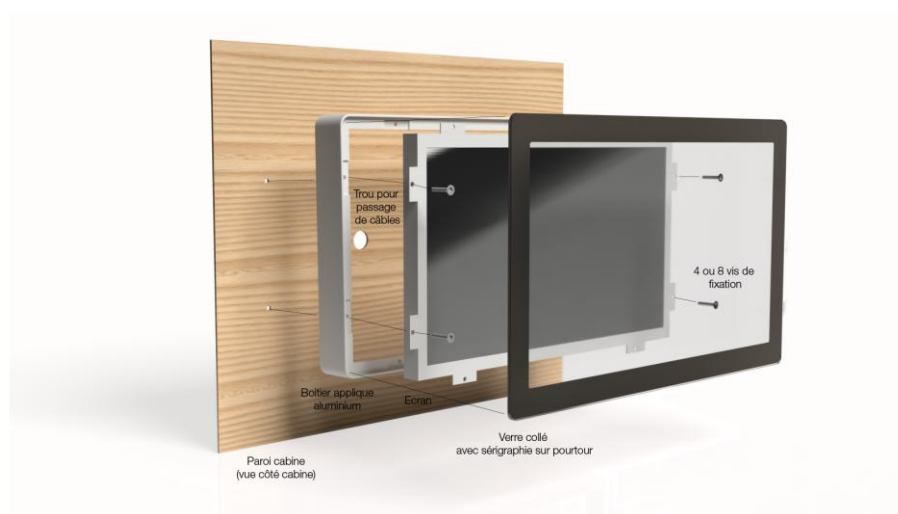
Schéma d'implantation d'un écran finition en applique
