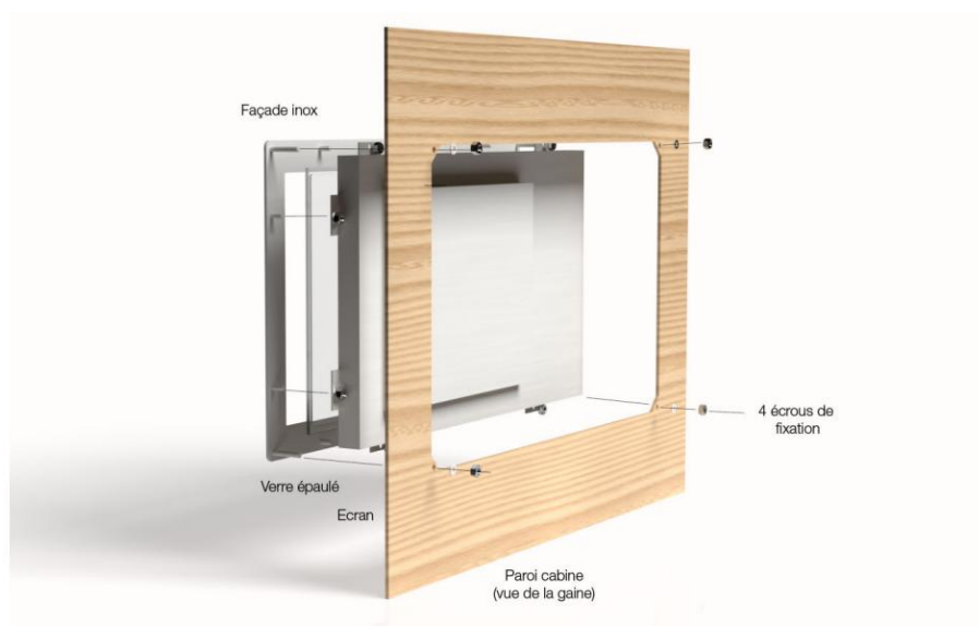
Schéma de montage écran SPOTLOOK finition façade inox (vue côté gaine ascenseur)
