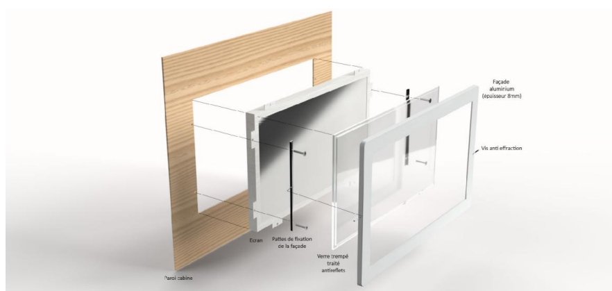
Schéma de principe de l'installation de l'écran cabine avec façade alu vissée
